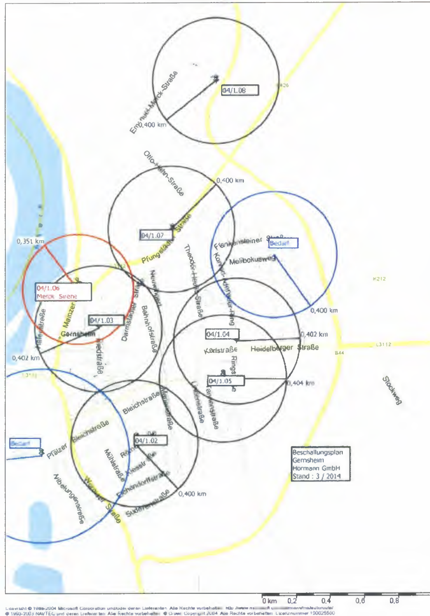
Anlage: Beschallungsplan
