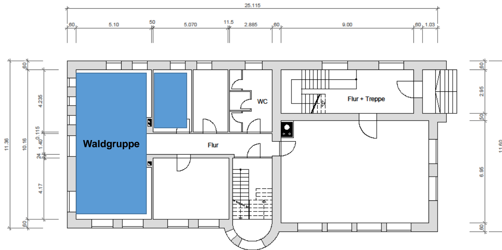
ERDGESCHOSS M 1:100
