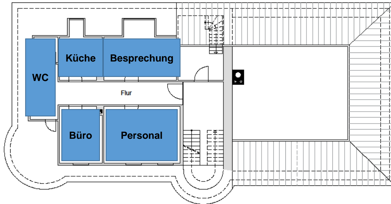
DACHGESCHOSS M 1:100
