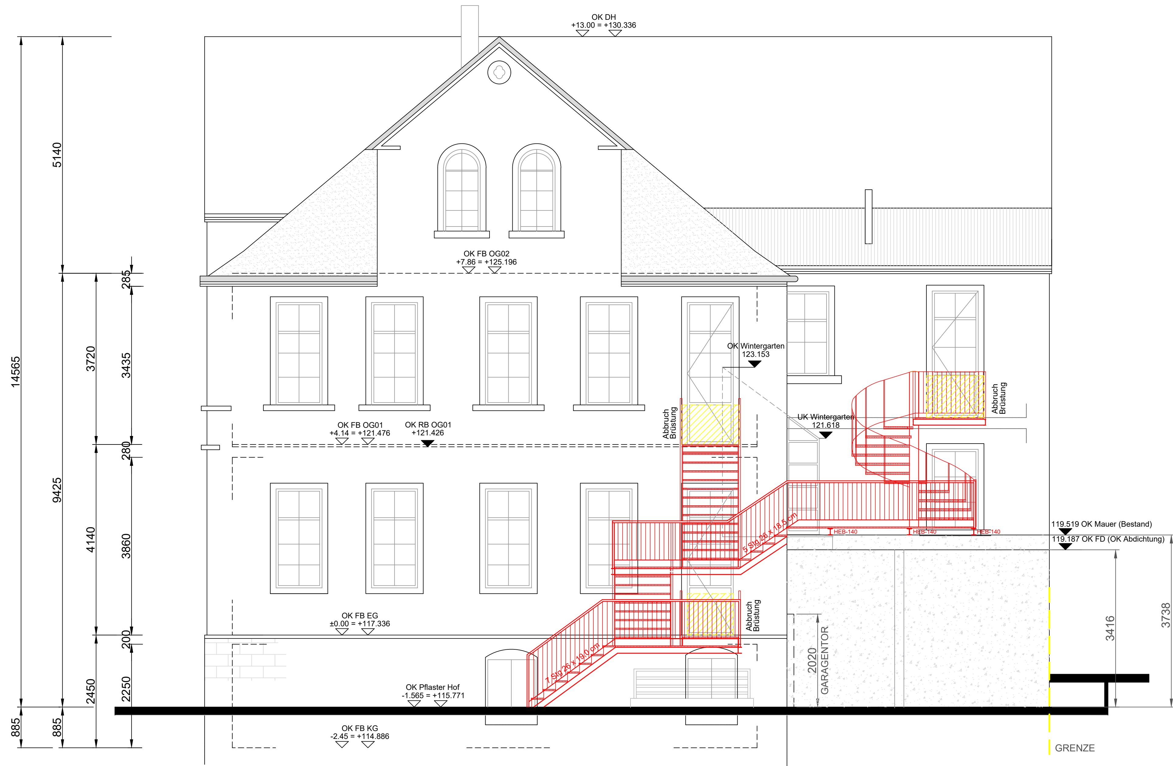
NORDANSICHT
