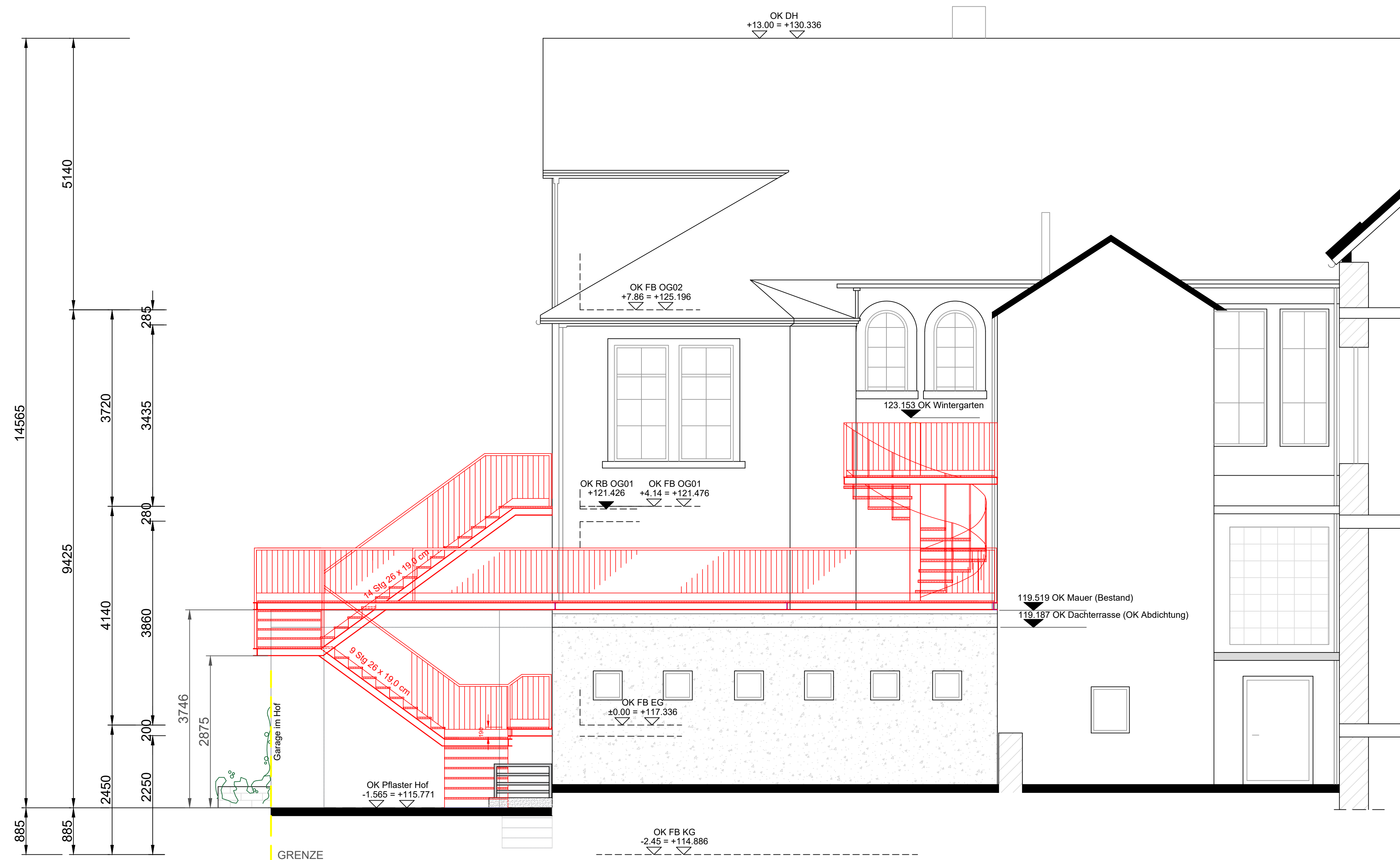
WESTANSICHT
