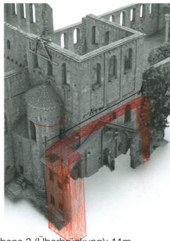
Ebene 3 (Überbrückung): 11m, (UK Träger ~10m)
