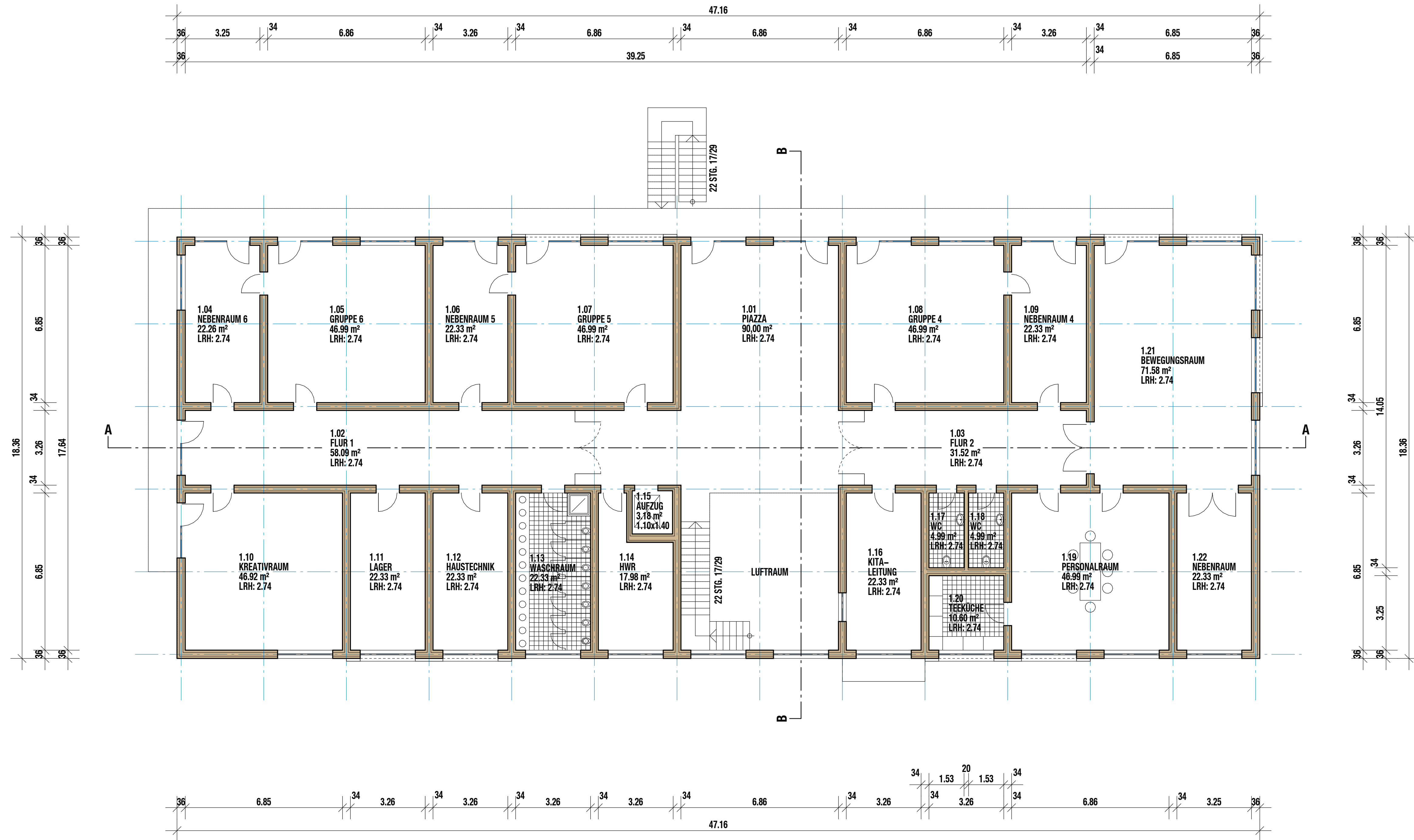
OBERGESCHOSS M. 1:100
