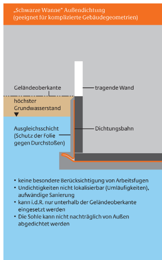
Abbildung 23: systematischer Aufbau Schwarze Wanne
