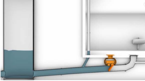
Abbildung 25: Rückstauverschluss
