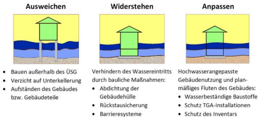
Abbildung 8: Hochwasserschutzstrategien der Bauvorsorge
