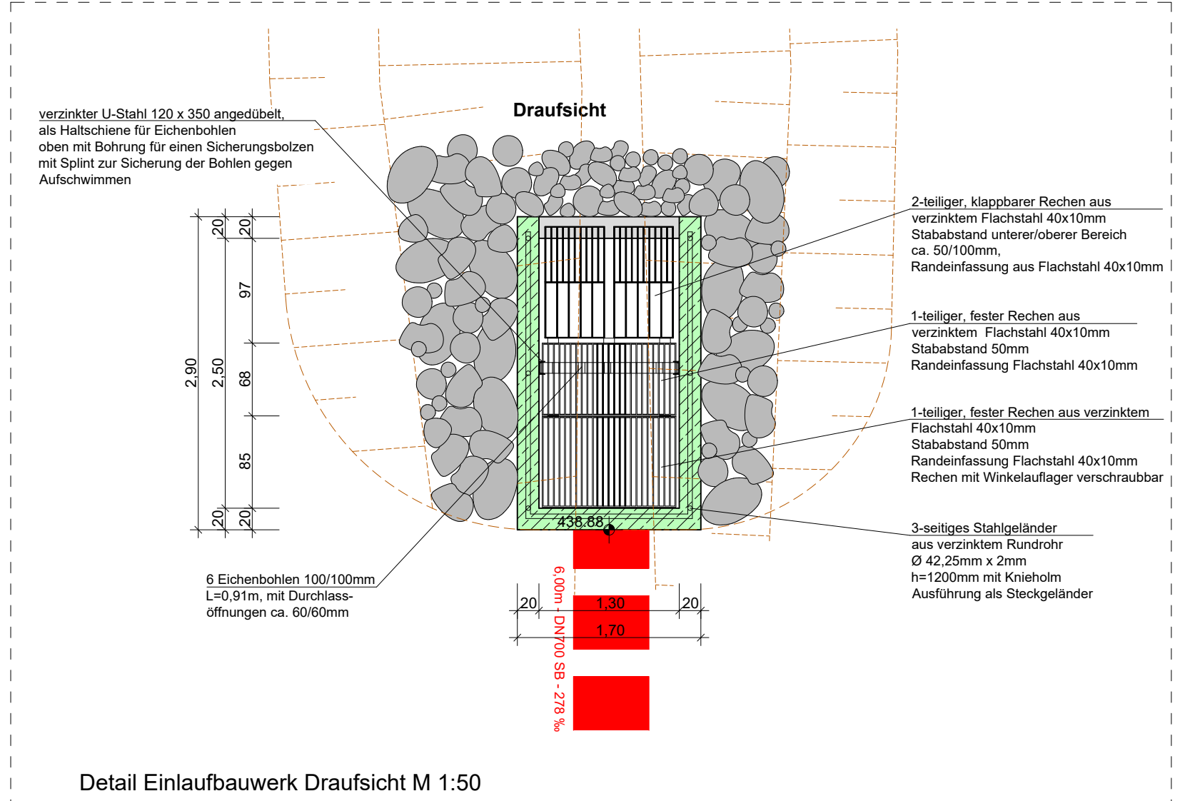
Detail Einlaufbauwerk Draufsicht M 1:50
