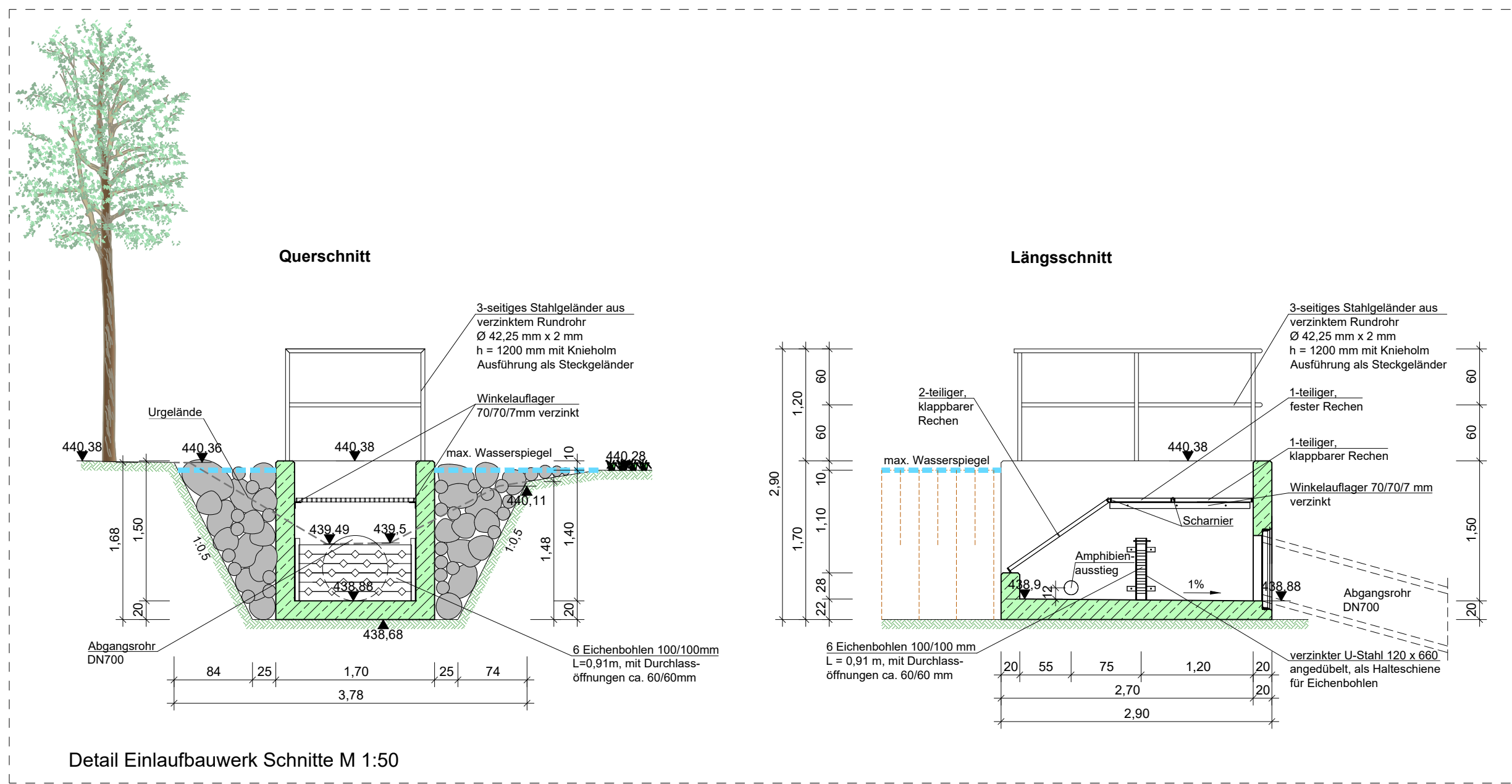
Detail Einlaufbauwerk Schnitt M 1:50
