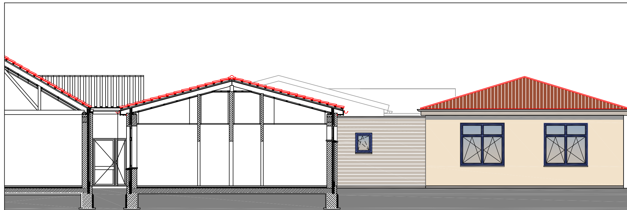
Ansicht West M 1:50
