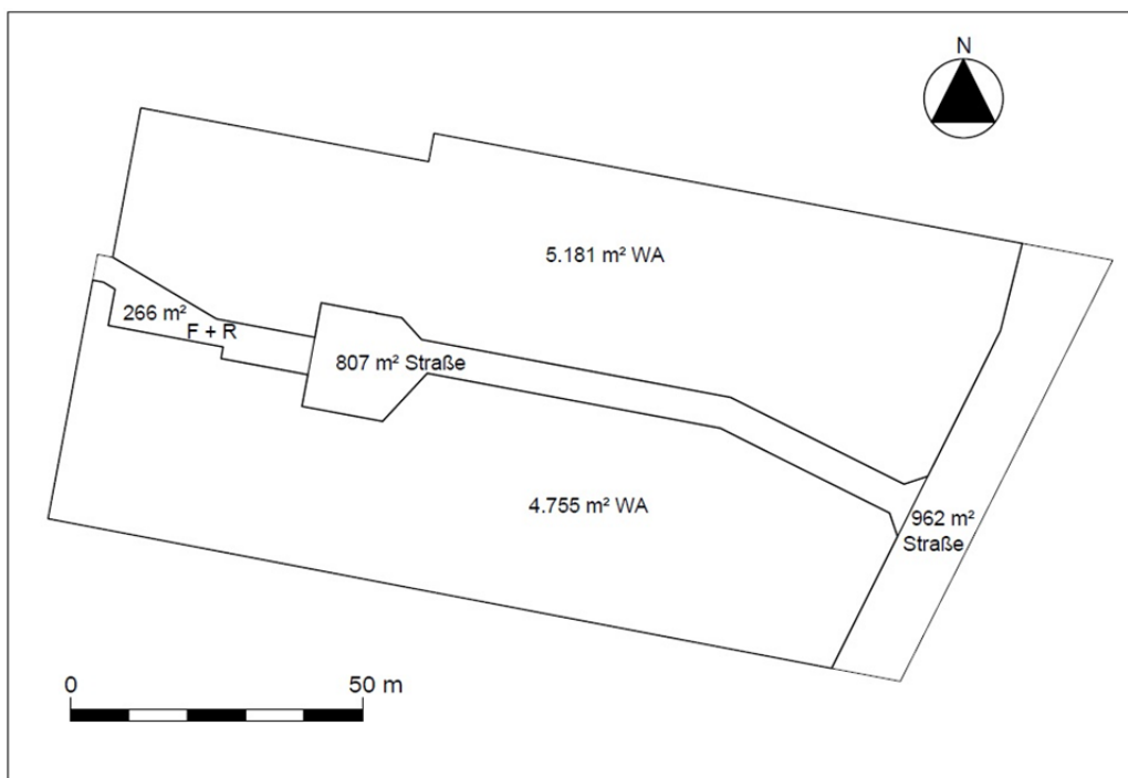
Flächenübersicht Planung
