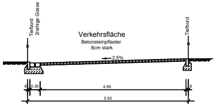
Schnitt (B-B) (Maßstab 1:50)
