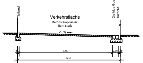
Schnitt (A-A) (Maßstab 1:50)
