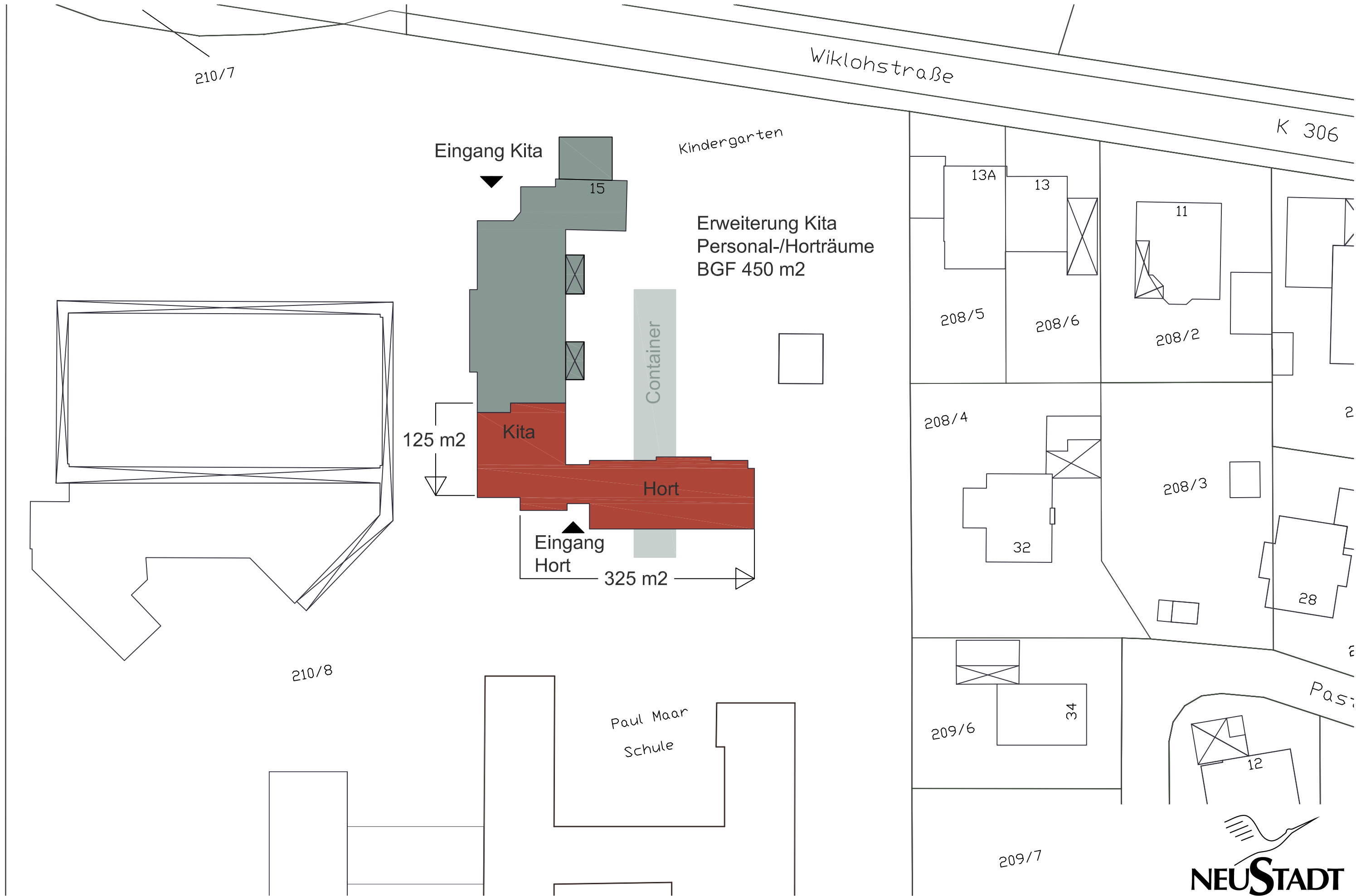
KITA Mandelsloh - Erweiterung Sozialräume und Hortgruppen - Lageplan M 1:500
