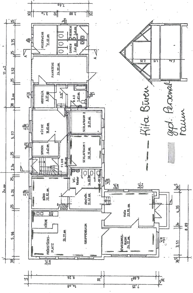
ERDGESCHOSS-GRUNDRISS
