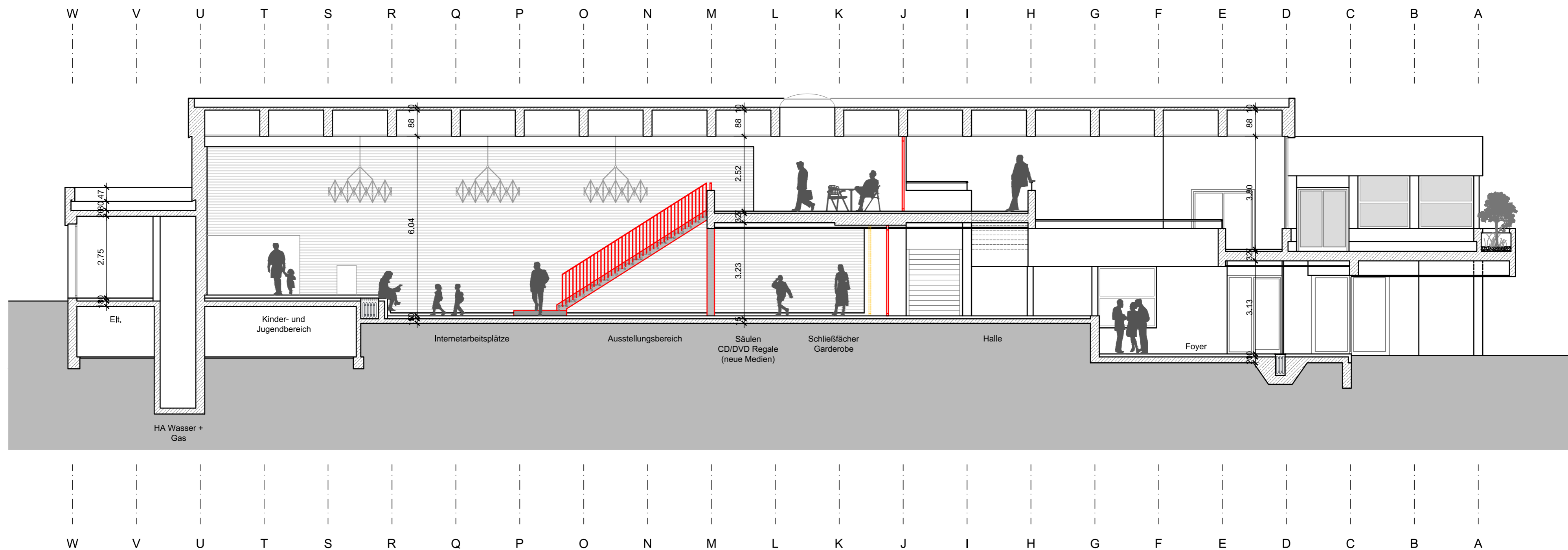
Schnitt A-A M 1:100
