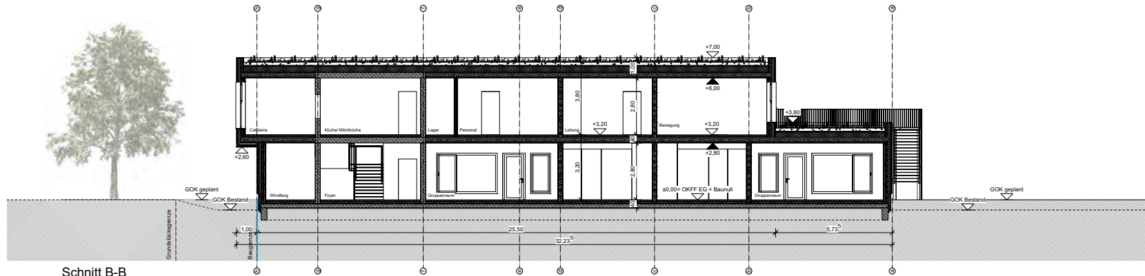
Schnitt B-B
