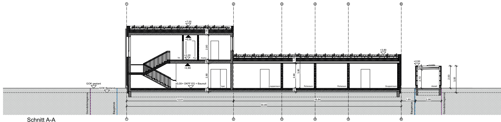
Schnitt A-A
