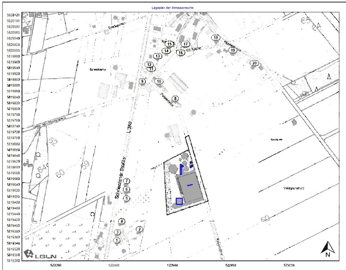
Abb. 10: Lageplan der Immissionsorte im Umfeld der Biogasanlage Maßstab 1 : ~7.500
