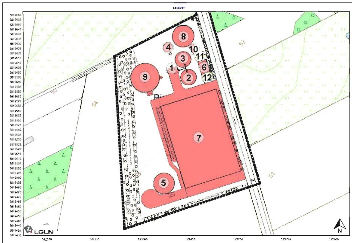
Abb. 2: Lageplan der Biomasseanlage „Resserithe“ der Biogas Schneeren GbR. Maßstab 1 : ~ 2.300
