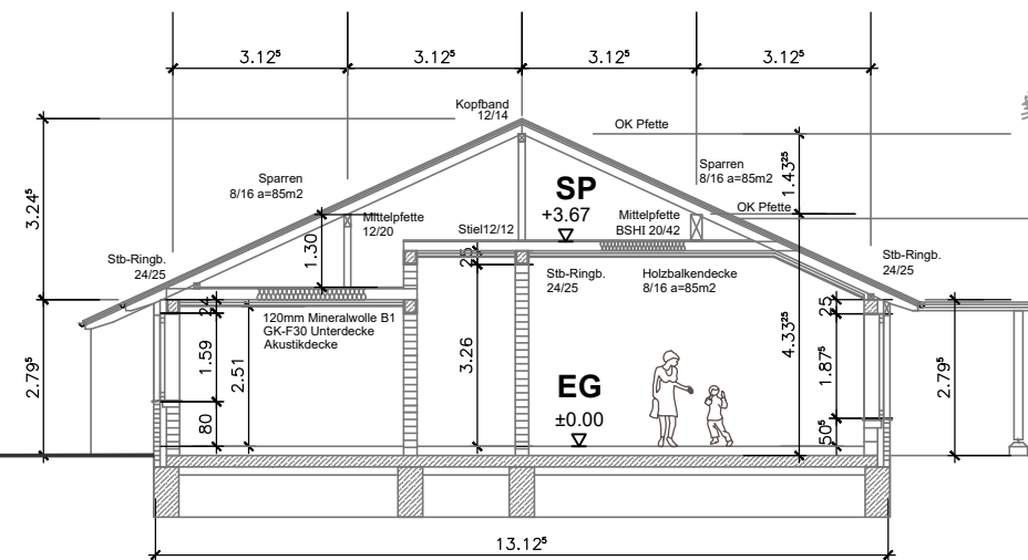
Schnitt Bestand
