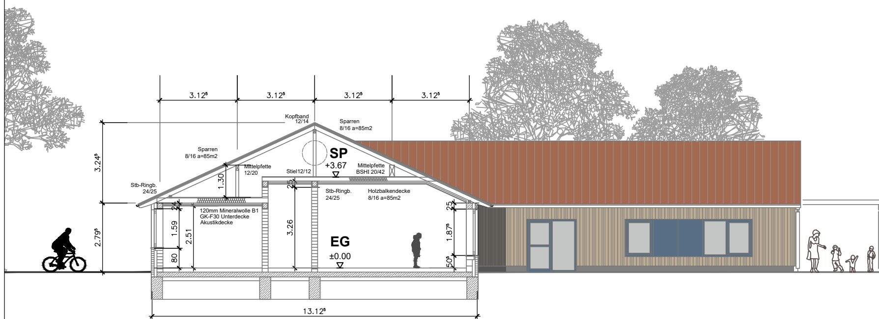
SCHNITT 1
