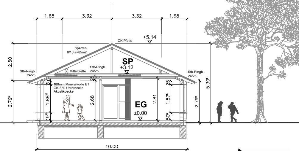
Schnitt 2
