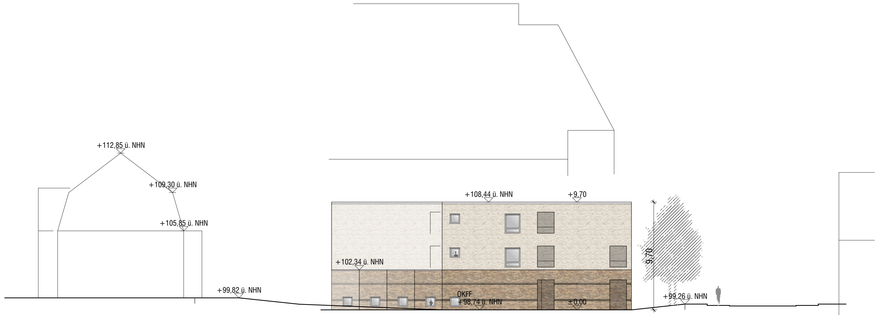
Ansicht Süden
