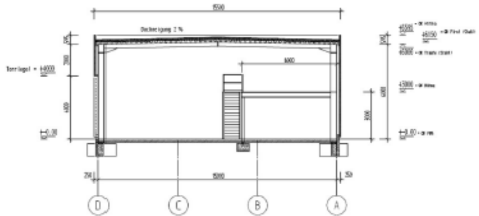
Querschnitt
