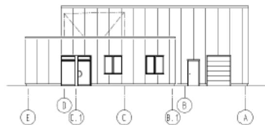
Ansicht Achse 1
