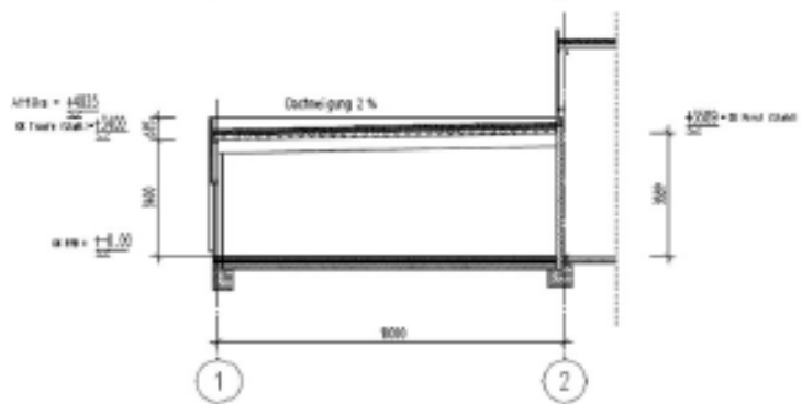
Schnitt 1 - 1
