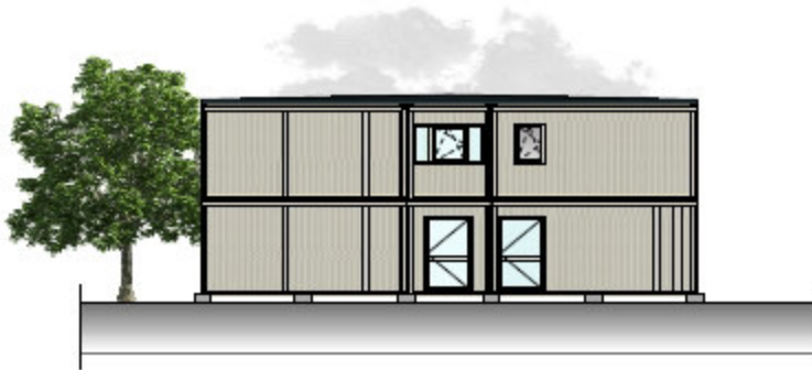
Ansicht 2 M.: 1:100
