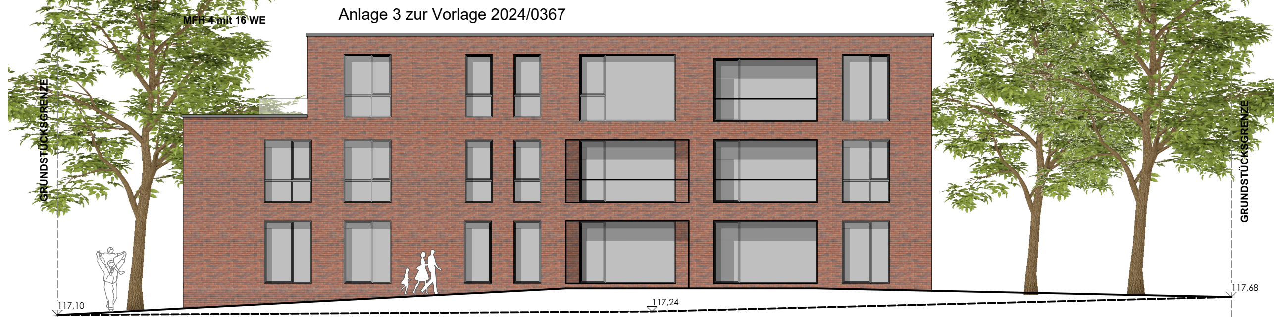
ANSICHT SÜD_OST
