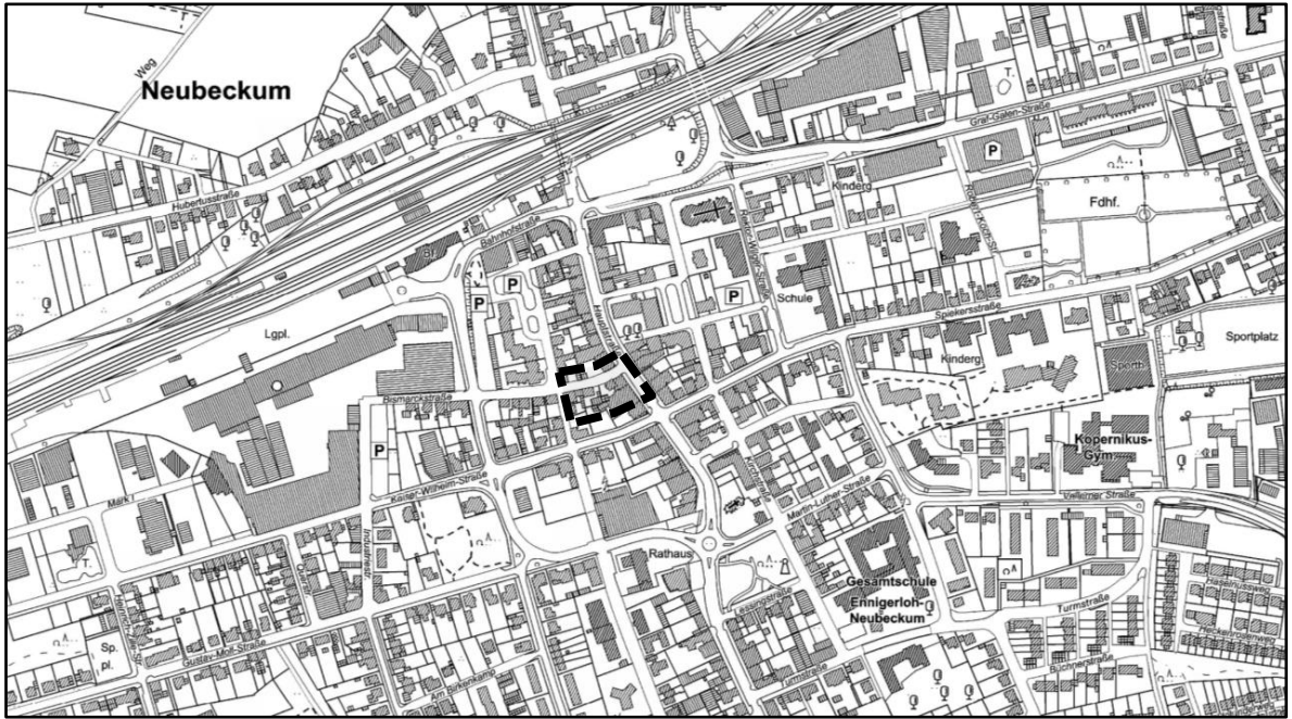
Abbildung 1: Räumliche Geltungsbereiche des Bebauungsplanes Nr. N20 „Mauerstraße/Hauptstraße/Kaiser-Wilhelm-Straße, 1. Änderung
