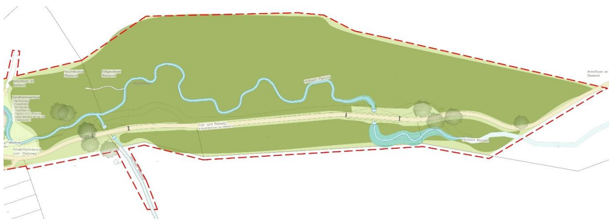
Abb. 2: Geplante Maßnahmen zum Abschnitt Auenwald (Lageplan – Nr. 3.04)
